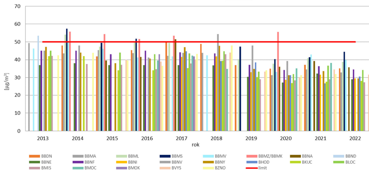
Obr. 24: Vývoj 36. nejvyšších denních koncentrací PM 10 za kalendářní rok, 2013–2022
