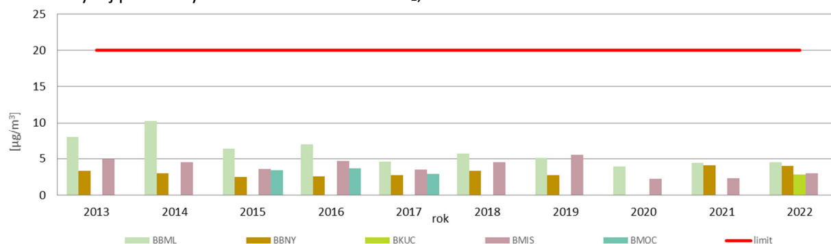
Obr. 31: Vývoj průměrných ročních koncentrací SO 2 , 2013–2022
