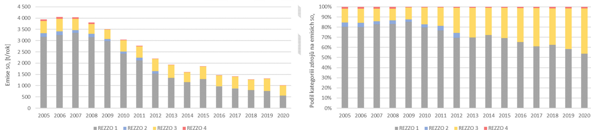
Obr. 8: Vývoj emisí a podílů kategorií REZZO 1-4 na celkových emisích SO x , Jihomoravský kraj, 2005-2020
