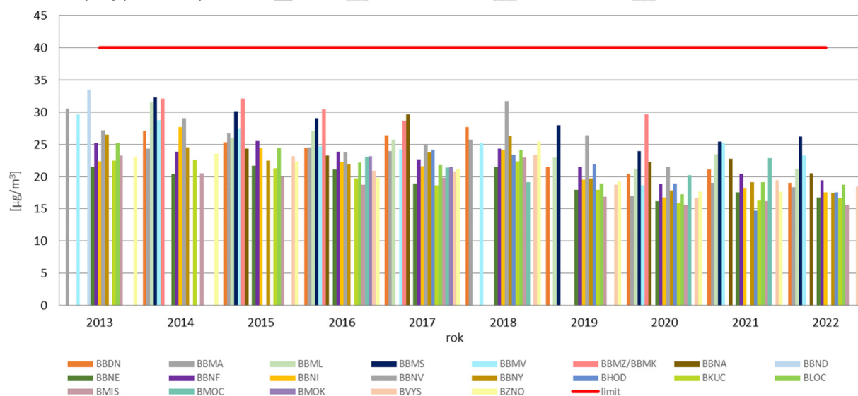
Obr. 23: Vývoj průměrných ročních koncentrací PM 10 , 2013–2022
