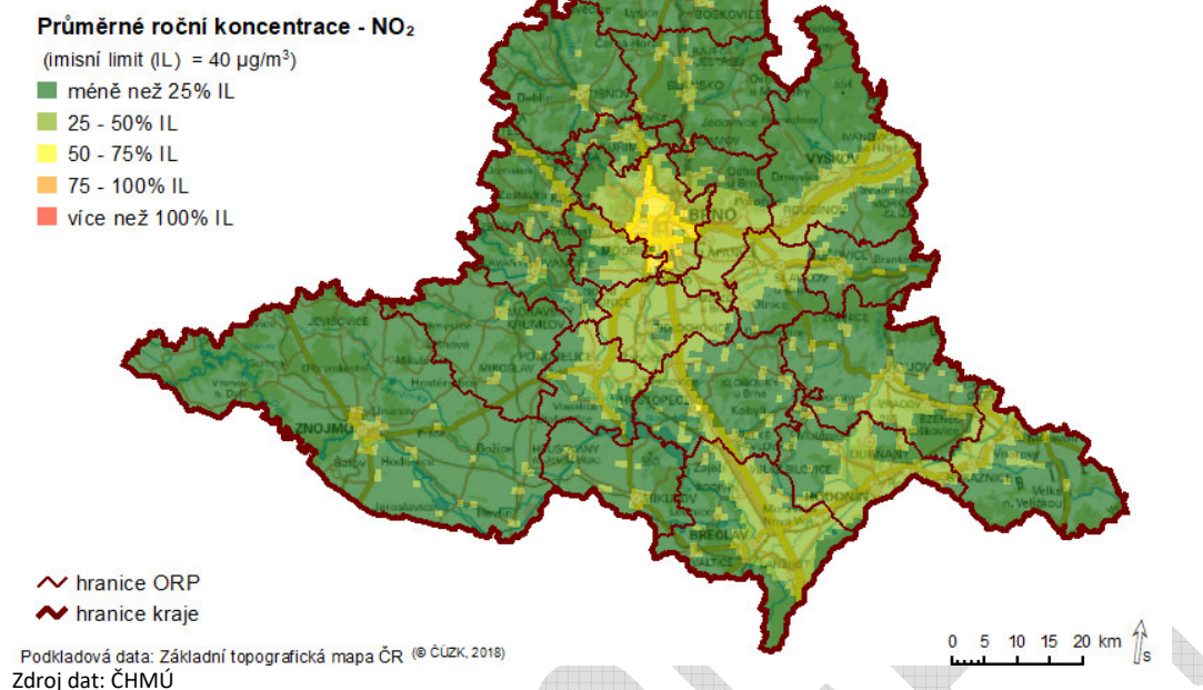
Obr. 12: Pětileté průměry 2017-2021, průměrné roční koncentrace NO 2 , Jihomoravský kraj Pětileté průměrné koncentrace 2017-2021 Jihomoravský kraj
