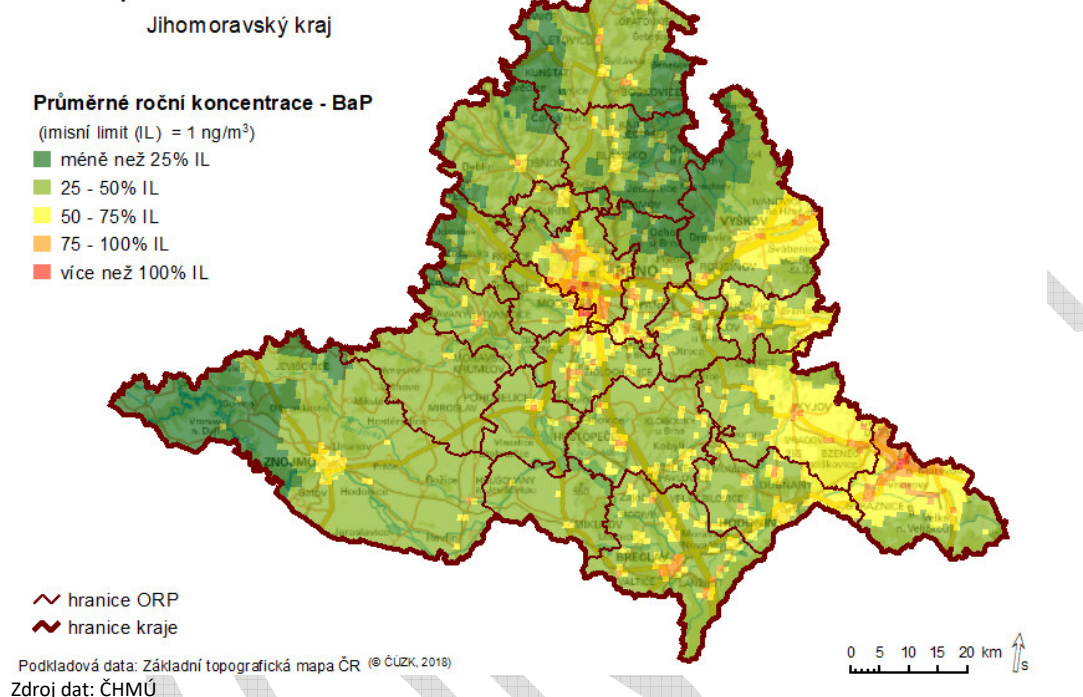
Obr. 17: Pětileté průměry 2017-2021, průměrné roční koncentrace BaP, Jihomoravský kraj Pětileté průměrné koncentrace 2017-2021
